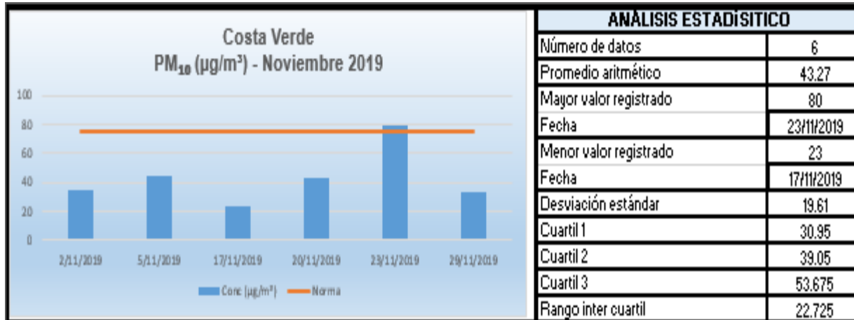
Gráfica 9. Monitor Costa Verde. Noviembre de 2019
