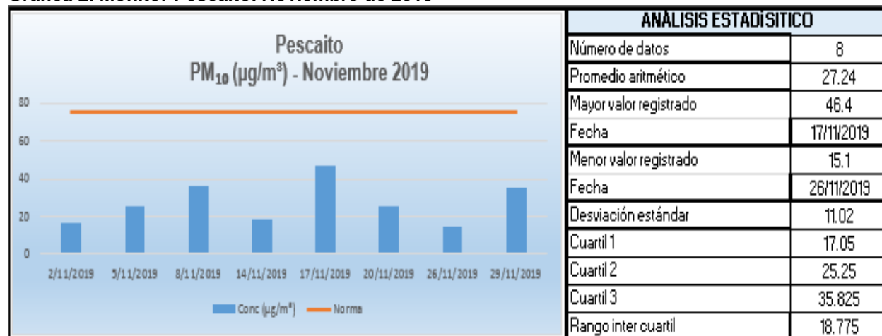
Gráfica 2. Monitor Pescaito. Noviembre de 2019
