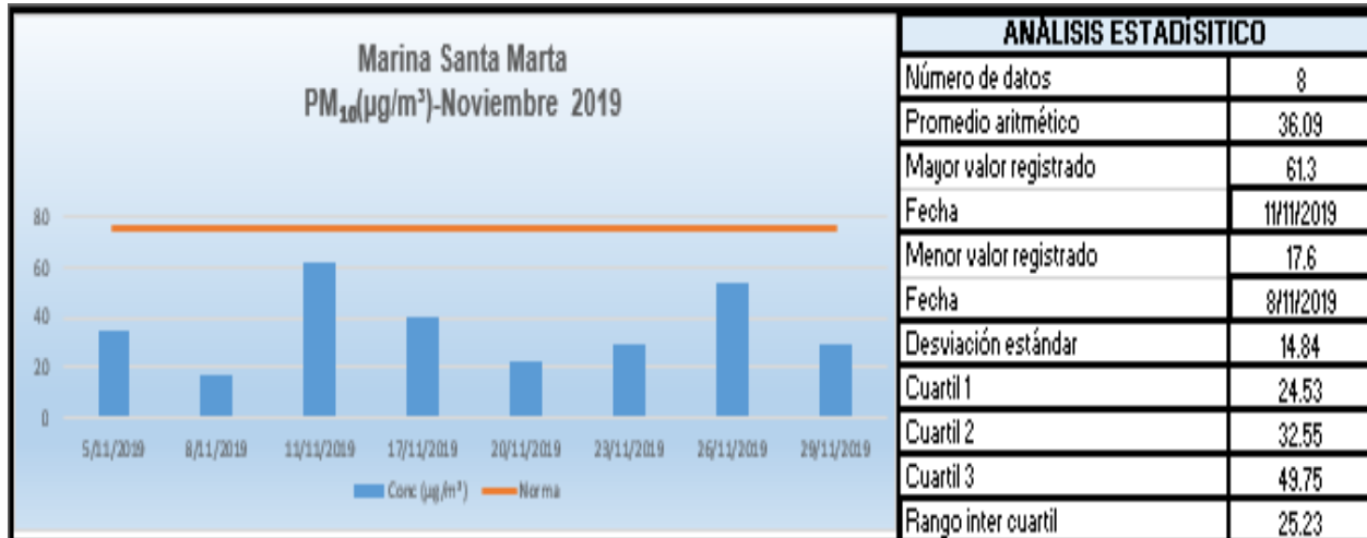
Gráfica 3. Monitor Marina Santa Marta. Noviembre de 2019
