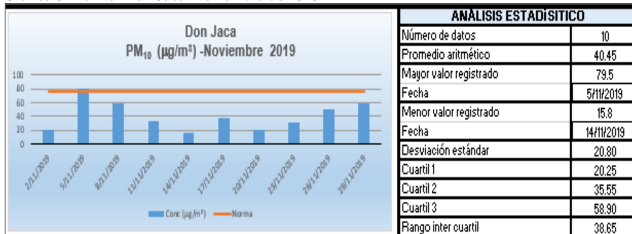
Gráfica 5. Monitor Don Jaca. Noviembre de 2019
