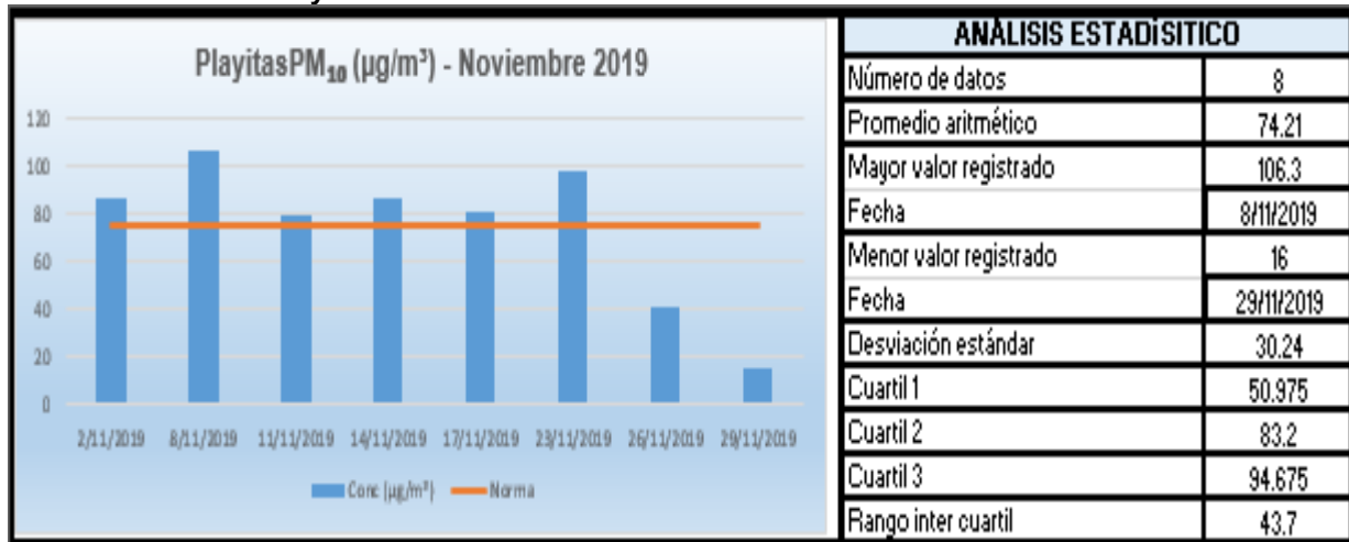
Gráfica 8. Monitor Playitas. Noviembre de 2019
