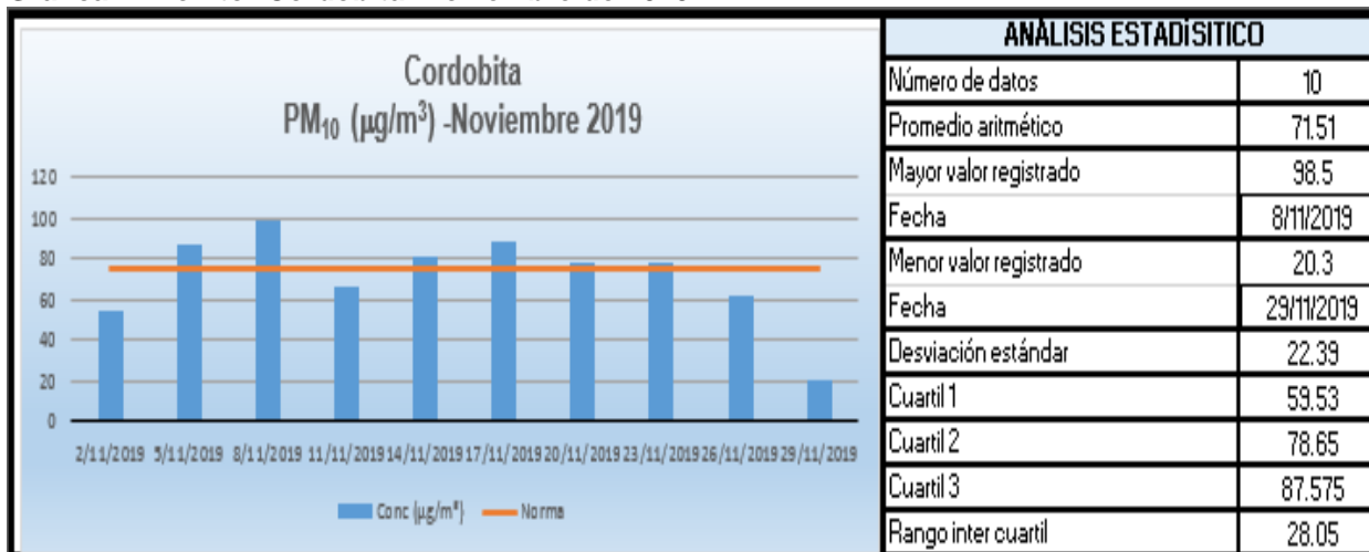
Gráfica 7. Monitor Cordobita. Noviembre de 2019
