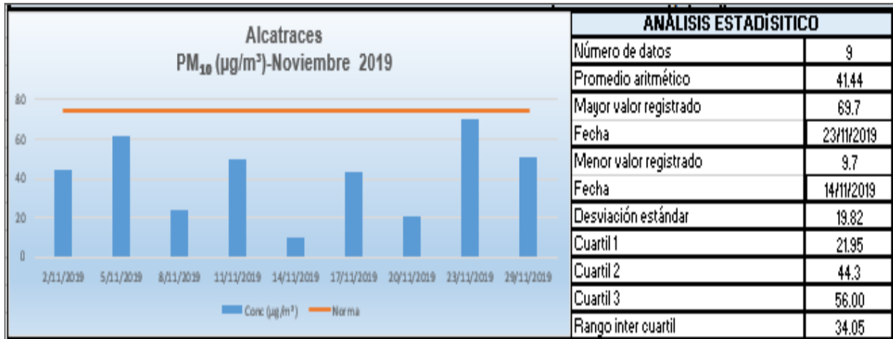
Gráfica 6. Monitor Alcatraces. Noviembre de 2019
