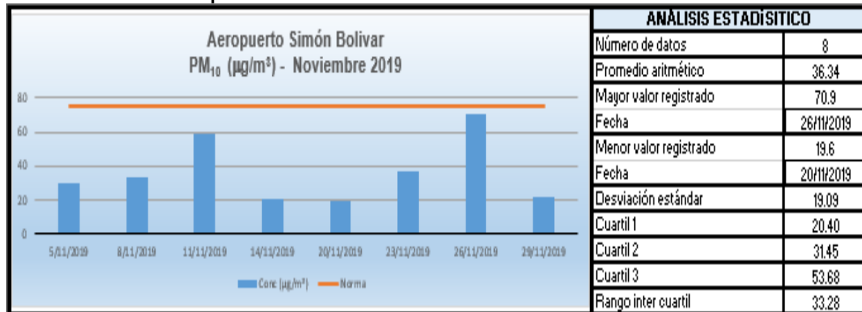
Gráfica 4. Monitor Aeropuerto. Noviembre de 2019
