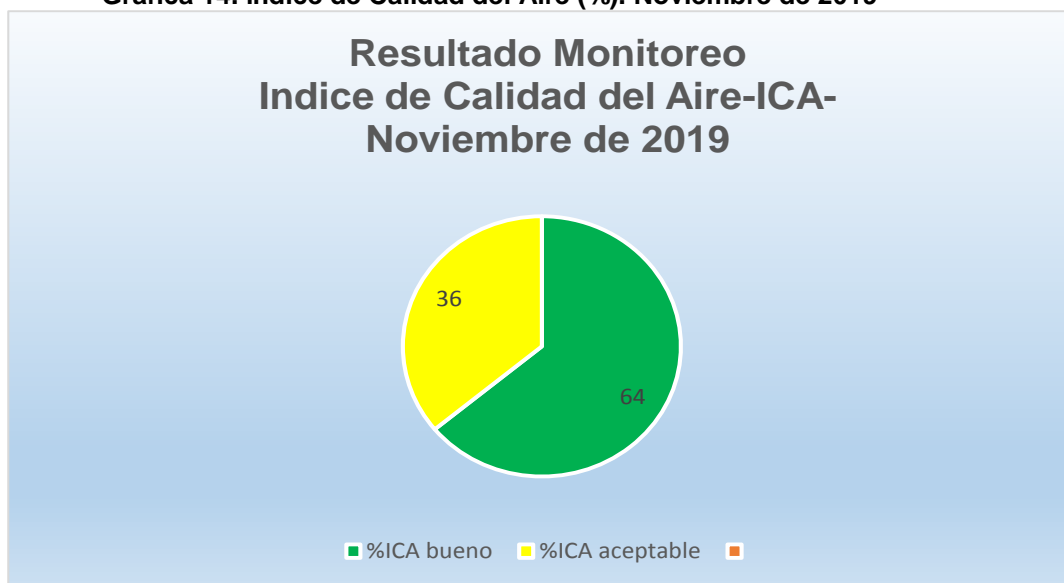
Gráfica 14. Índice de Calidad del Aire (%). Noviembre de 2019
