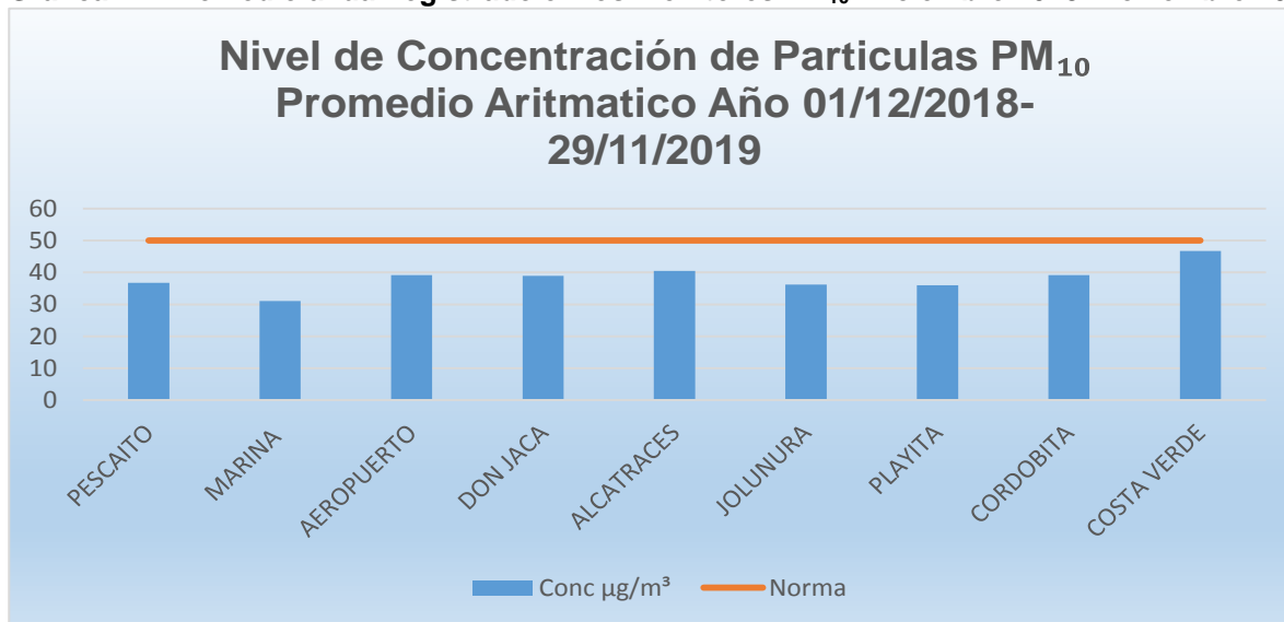
Gráfica 12. Promedio anual registrado en los monitores PM 10 . Diciembre 2018- Noviembre 2019
