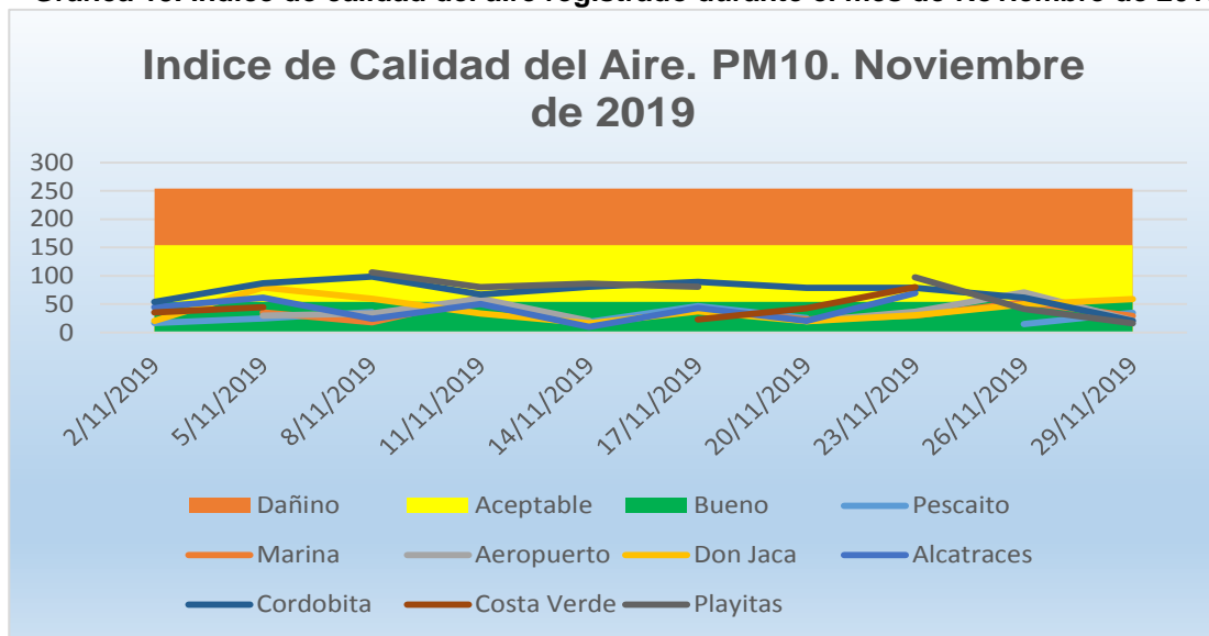
Gráfica 13. Índice de calidad del aire registrado durante el mes de Noviembre de 2019
