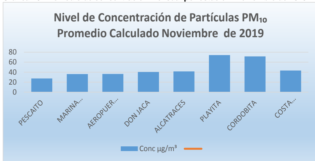
Gráfica 10. Promedio de concentración mensual por estación. Noviembre de 2019
