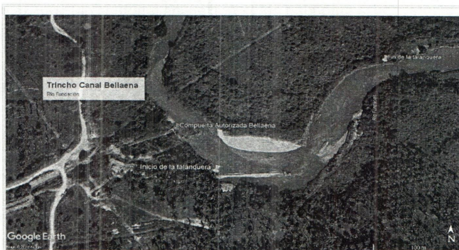
Figura 1. Trincho a lo largo y ancho del río Fundación en la bocatoma Bellaena (Elaboración propia. Google Earth). Coordenadas geográficas 10^{\circ}34'35.472''\text{N} - 74^{\circ}15'26.49''\text{O}
