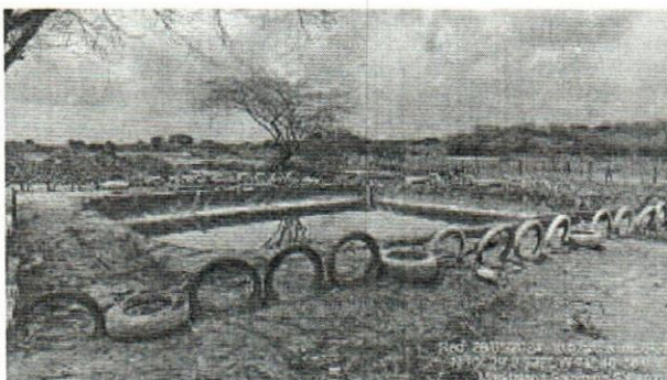
Fotografía No. 3. Piscina de lixiviados.
