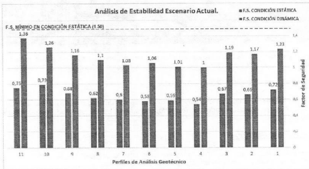
Figura 30. Resumen de factores de seguridad obtenidos para el análisis de estabilidad en el escenario actual.
