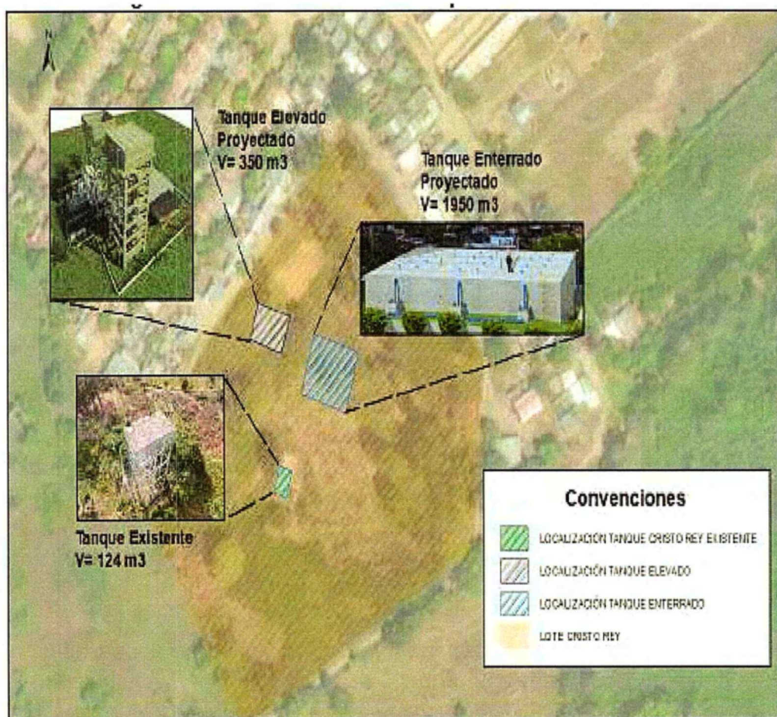
Ilustración 5 Localización de los tanques de almacenamiento.
