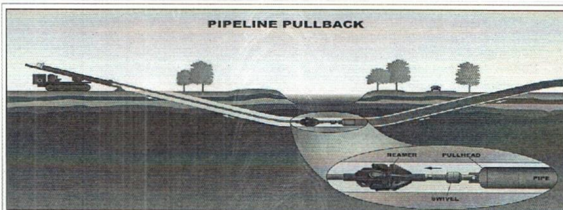
Figura 3. Esquema cruce utilizando método PHD. Fuente: Adaptado información técnica aportada por usuario
