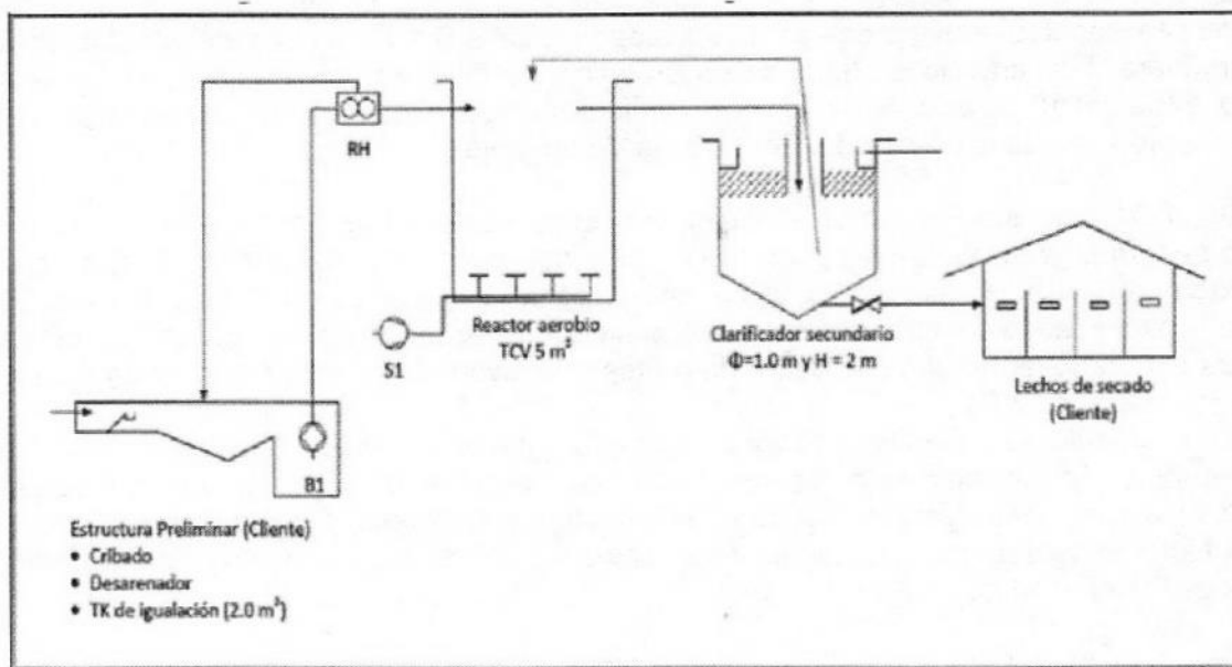
Diagrama de Aguas Residuales
