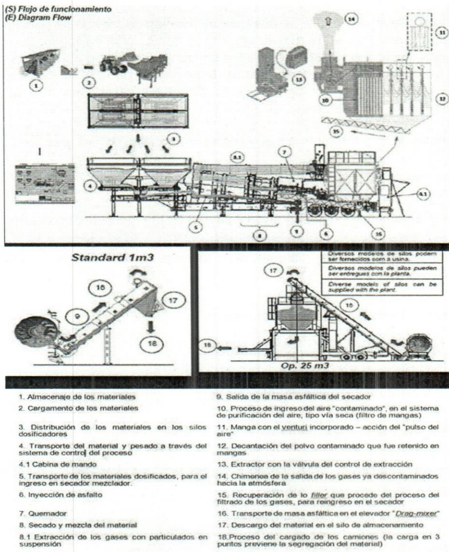
Gráfico 1: Diagrama de flujo de planta móvil de asfalto en caliente.
