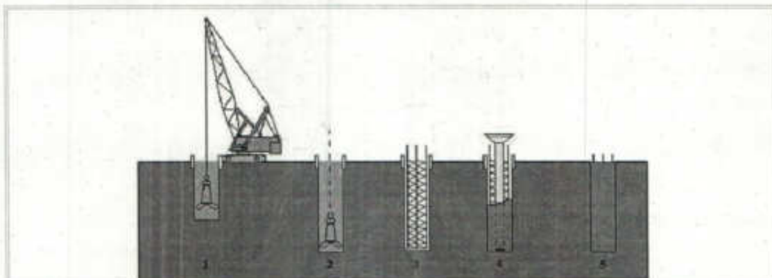
Figura 3. Construcción de pilotes TREMIE en zonas con nivel freático alto. Fuente: Procedimiento de construcción de cimentaciones y estructuras de contención. Yepes V (2020)
