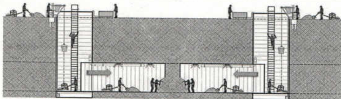
CORTE LONGITUDINAL POZOS DE LANZAMIENTO Y TUNNEL LINER
